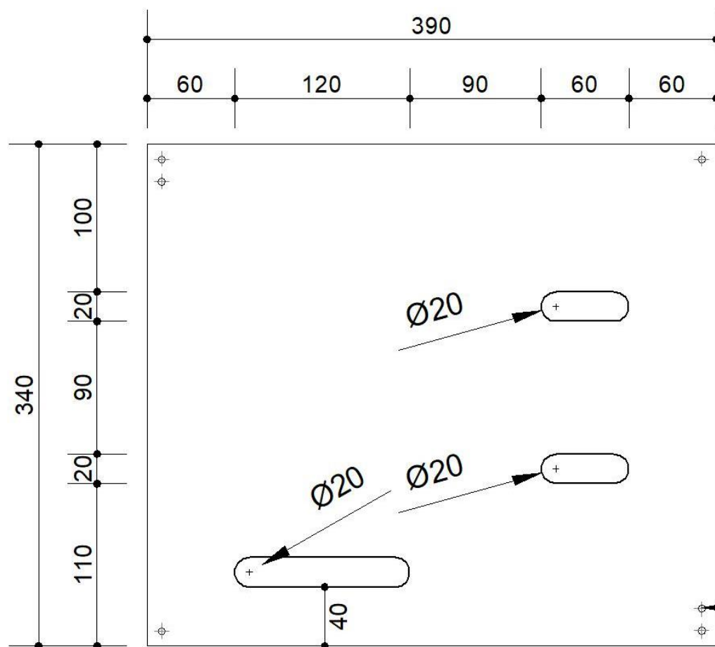
錶板開孔尺寸
