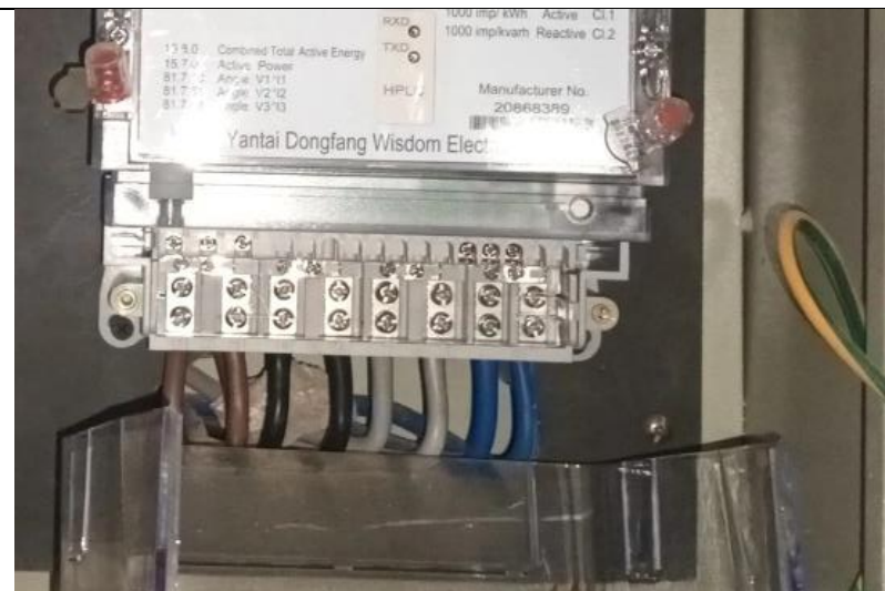
✓ 正確電錶接線排序及為正相序 (左至右: 棕、黑、灰、藍)
