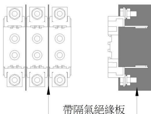
外露型熔斷器底座(帶隔氣絕緣板) 示意圖
