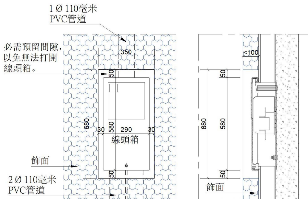
TYPE-A 線頭箱
