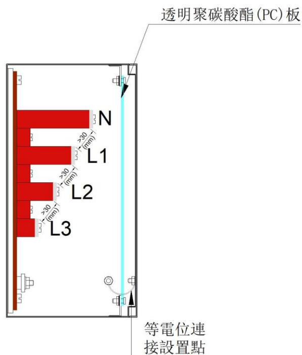
內部側視圖
