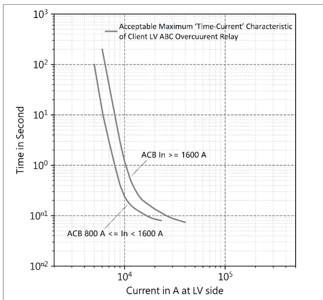
過流保護繼電器的最大時間 / 電流特性曲線
