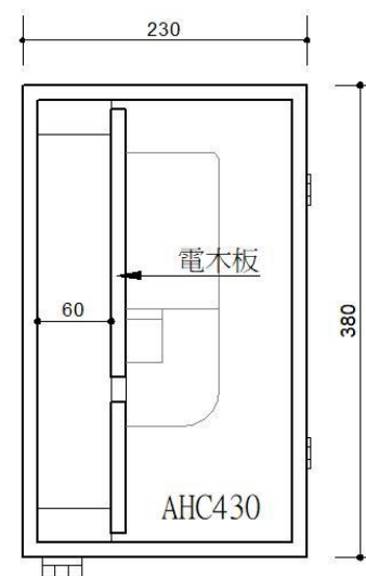
內部側視圖
