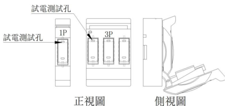
封閉型熔斷器底座示意圖
