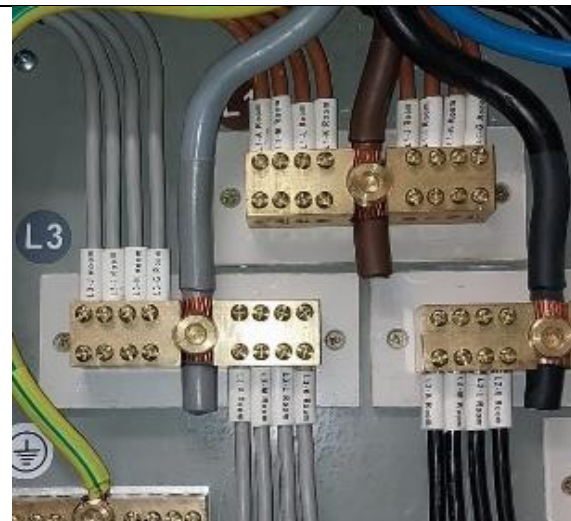
✓ 引入線的正確接駁方法
