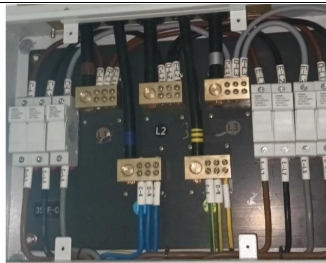
✓引入線必須有清楚易讀、耐用及適當的相位標示及單位識別標誌
