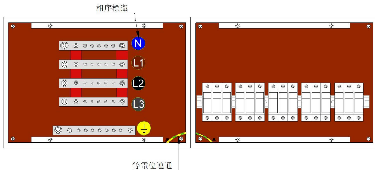
內部正視圖
