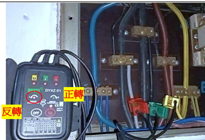
範例 26：✗ 電源相序錯誤(反轉)
