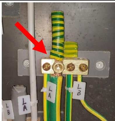
範例 29：✗上升總線與連接器(銅座)尺寸不匹配
