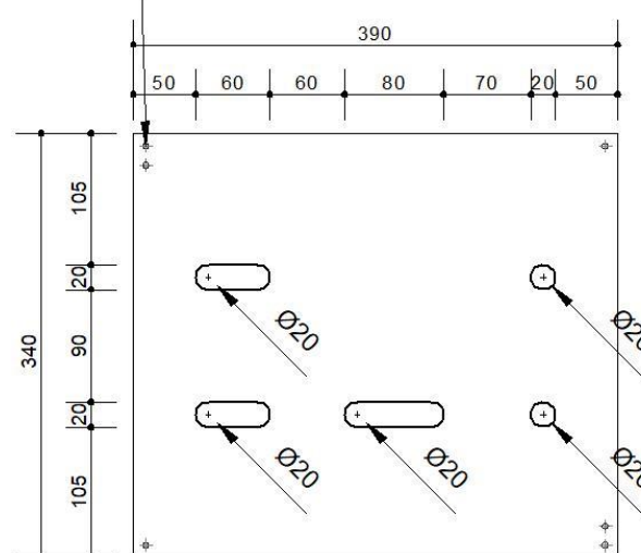
錶板開孔尺寸
