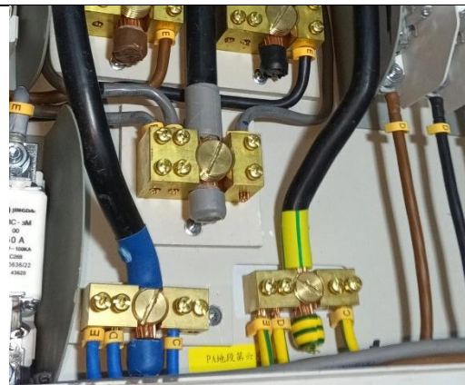
✓上升總線必須與銅座尺寸匹配
