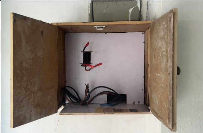
範例 19：✖ 電錶板未有使用電木板(Bakelite Plate)，開孔不符合規範， 沒有過江線
