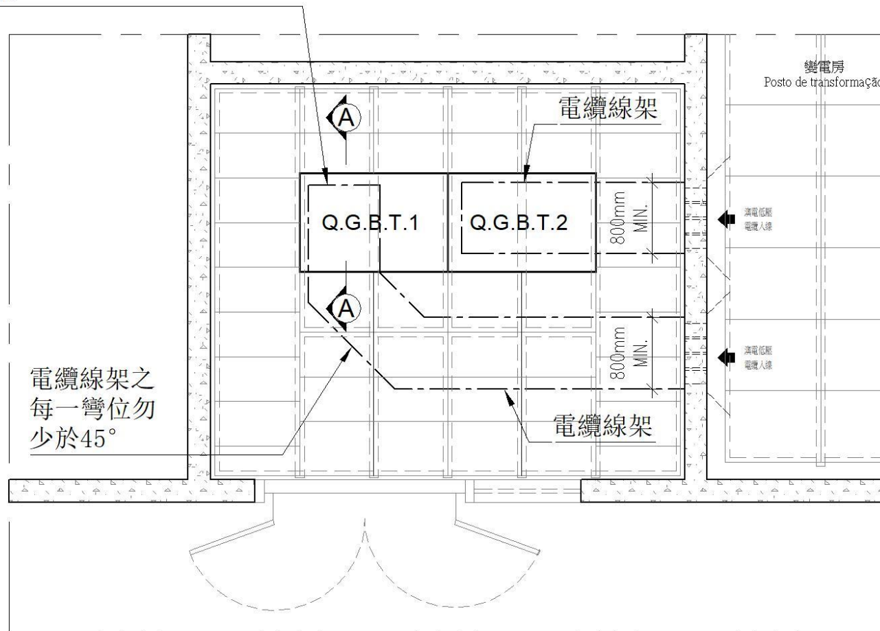
平面圖
