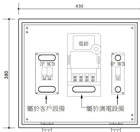
內部正視圖
