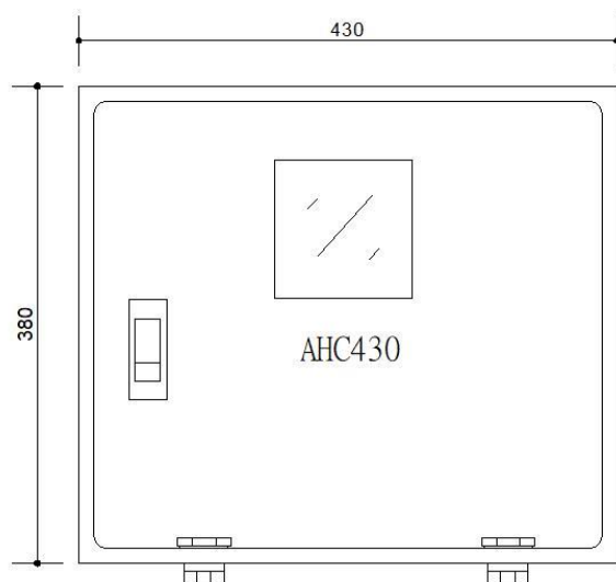
正視圖
