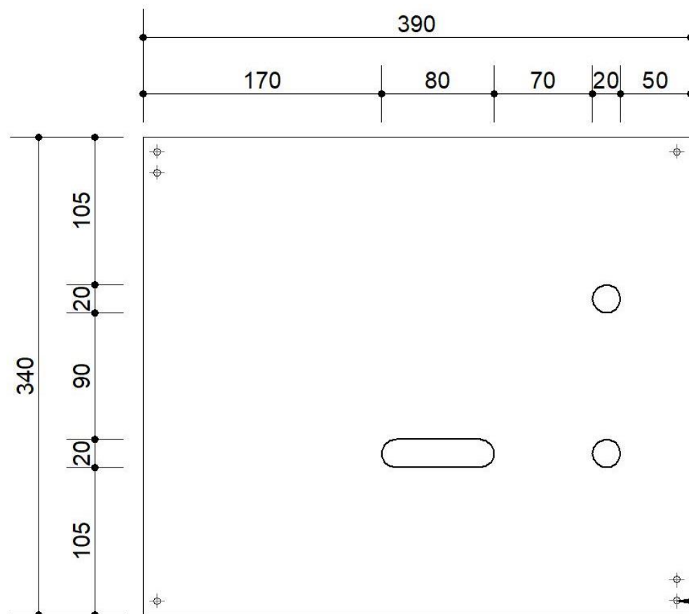
錶板開孔尺寸
